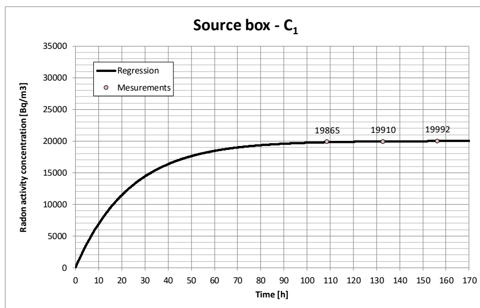
Figur 1 Radonkoncentration i primärlådan: uppmätt dygnsmedelvärde samt regressionskurvan.
