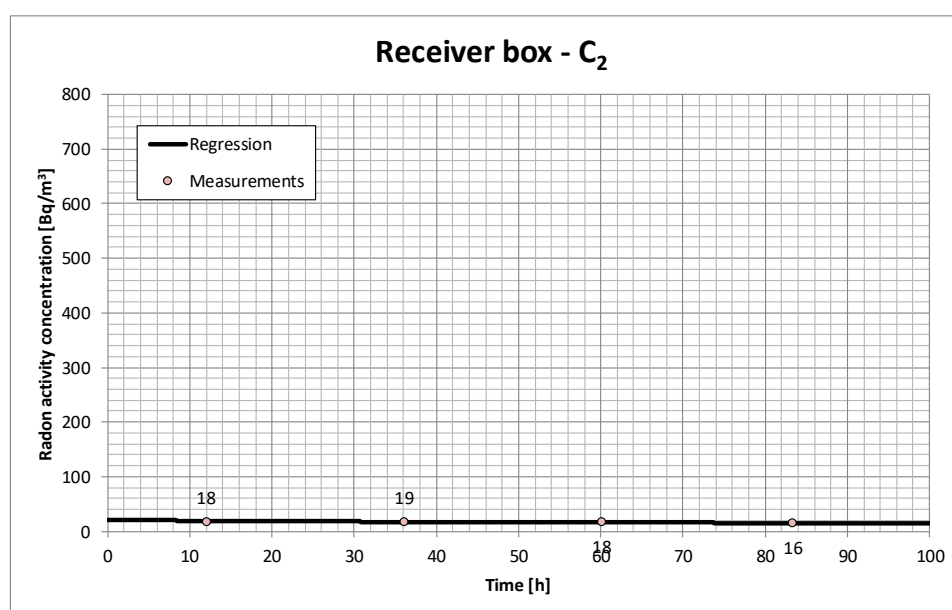
Figur 2 Radonkoncentration i sekundärlådan: uppmätt dygnsmedelvärde samt regressionskurvan.
